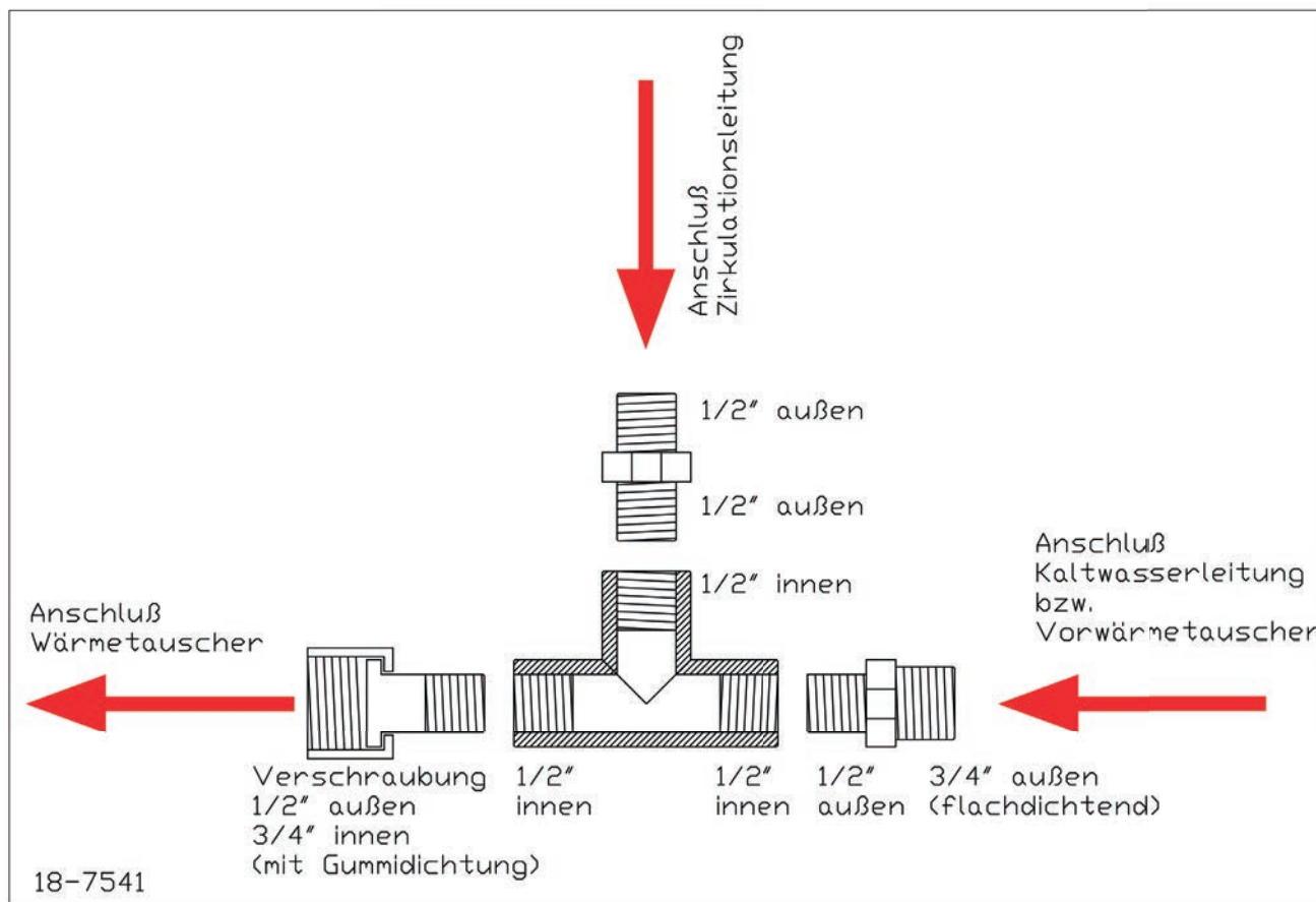
Abb. 1: Lieferumfang Zirkulationsanschluss (Fittings aus Messing)
